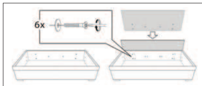
Montage Rückwand
