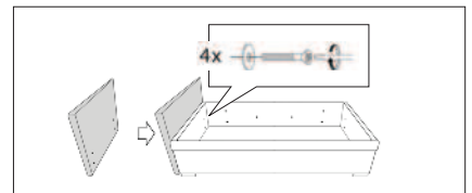
Montage Kopfteil, hier links analog rechts
